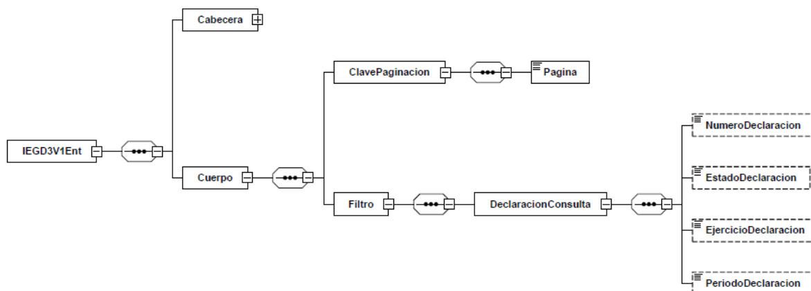
Figura 3: Cuerpo consulta
