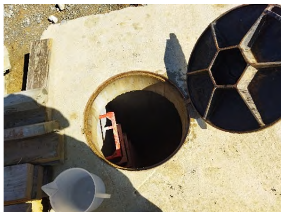
Foto nº26: Dren de fondo
