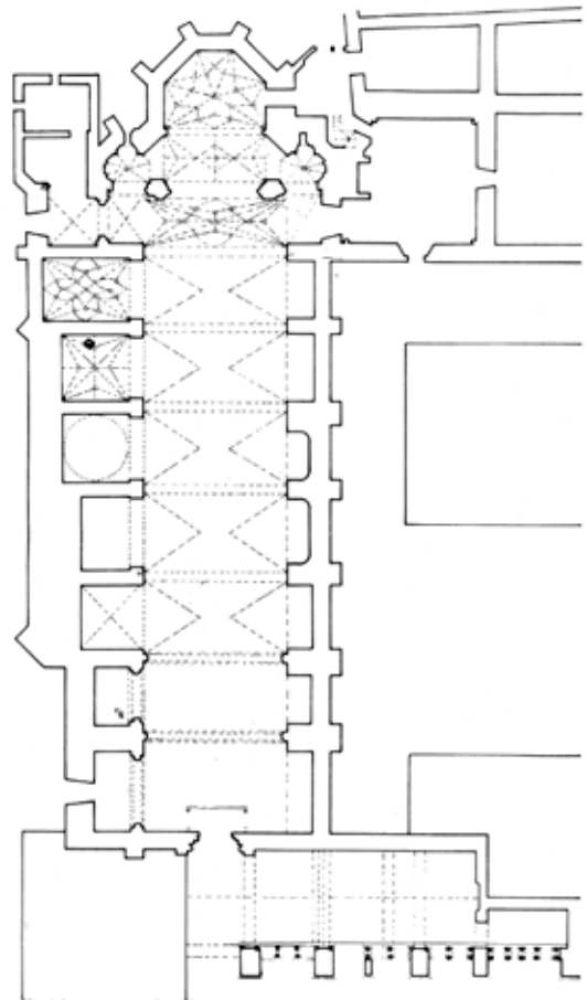
Figura 3. Planta de la iglesia del antiguo convento de San Francisco (sg. M. Millán y C. Sanz, tomado de Martínez, 1989: 94).
