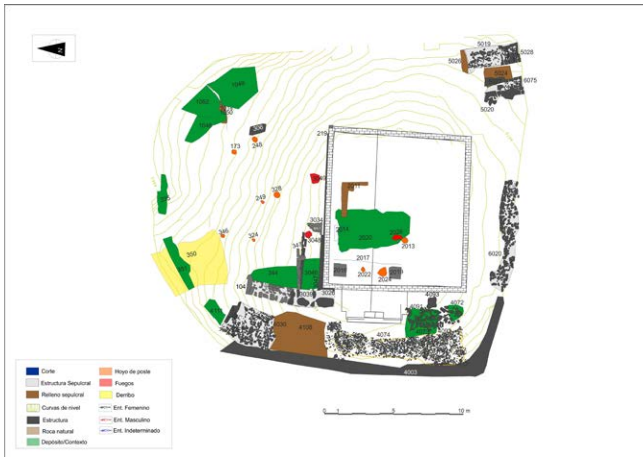
Figura 6. Plano de las estructuras atribuibles a la Fase 2. Ampliación (siglos XII-XIII).
