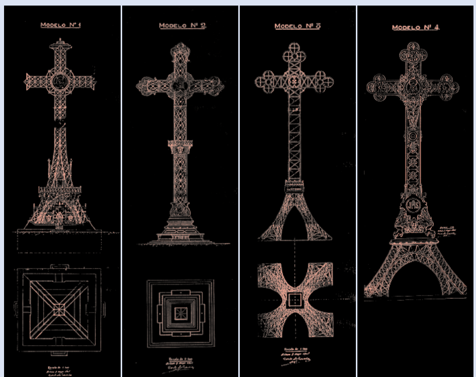
Los cuatro proyectos que diseñó Casto de Zavala para la cruz de Gorbeia y que ninguno fue su resultado (archivo AMV).
