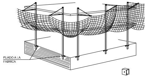
REDES PERIMETRALES CON SOPORTE METALICO _TIPO HORCA_
