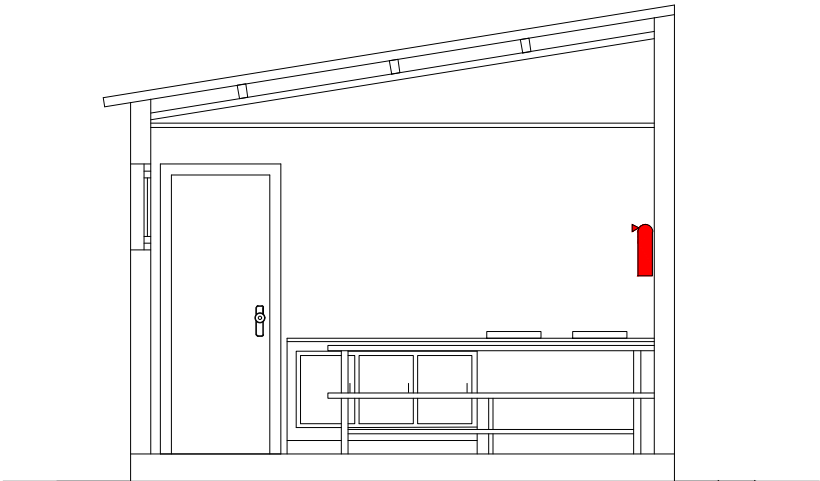
ASEO-VESTUARIOS-COMEDOR MÓDULO TIPO SECCIÓN A-B
