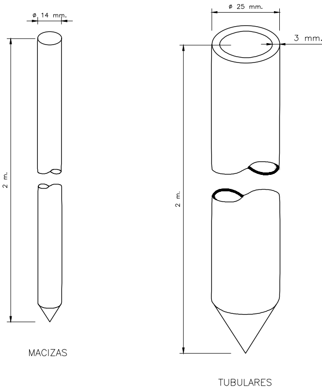
PICAS
