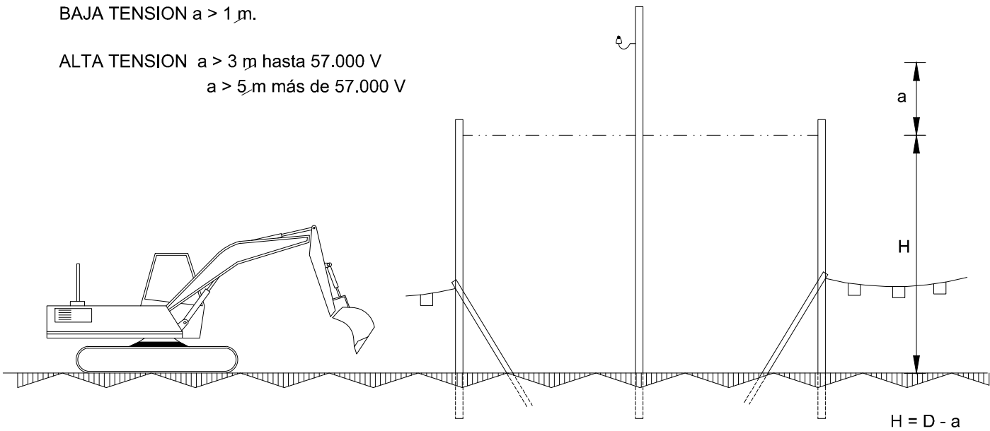
ALZADO LATERAL
