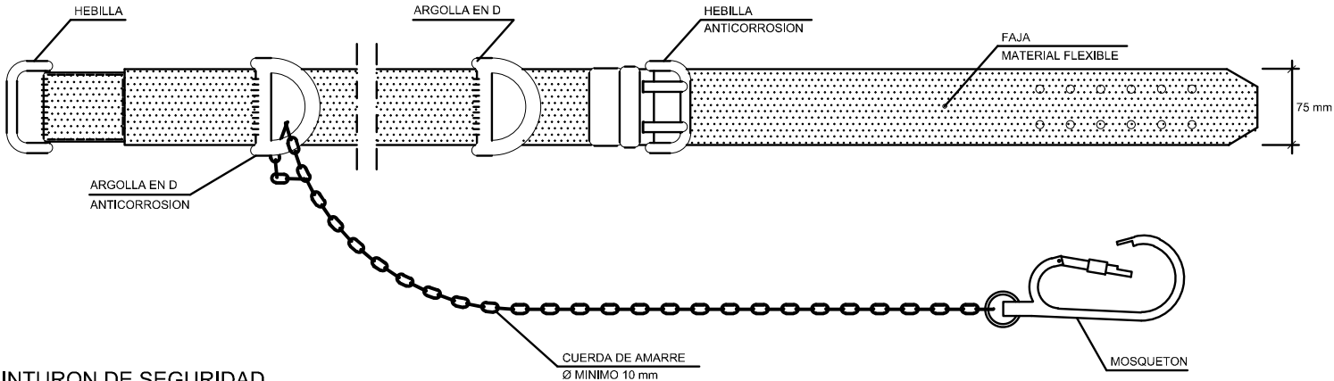
CINTURON DE SEGURIDAD CLASE A. TIPO 2
