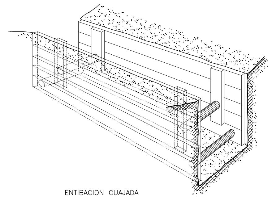
ENTIBACION CUAJADA
