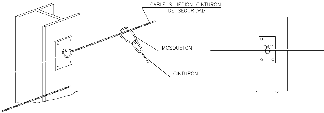
DETALLE SUJECCIÓN CINTURON DE SEGURIDAD
