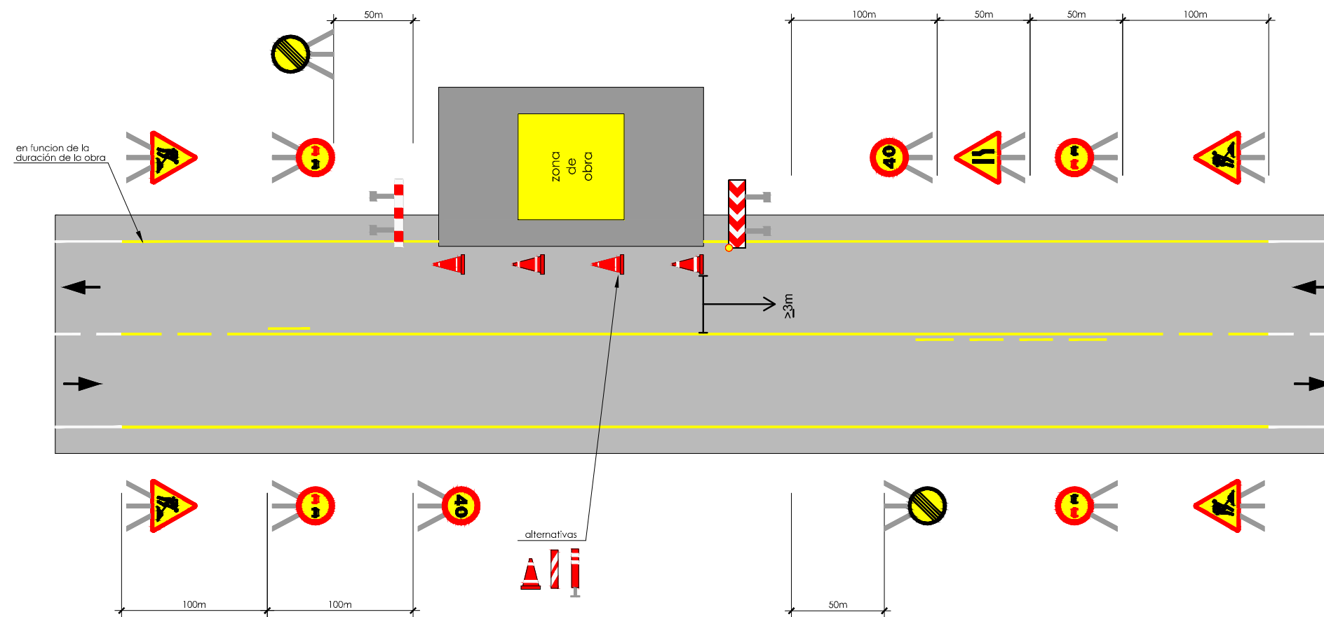
ZONA DE OBRA: en el arcén y parte del carril
