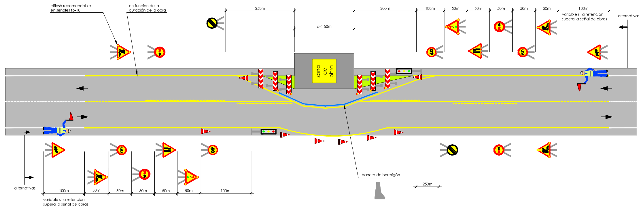
ZONA DE OBRAS: ocupando dos carriles
