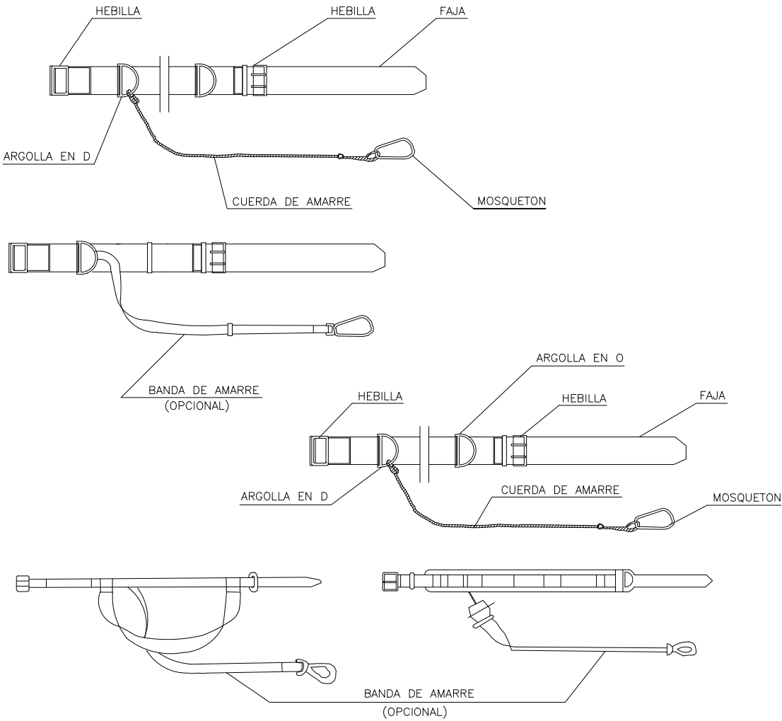
CINTURON TIPO – 1
