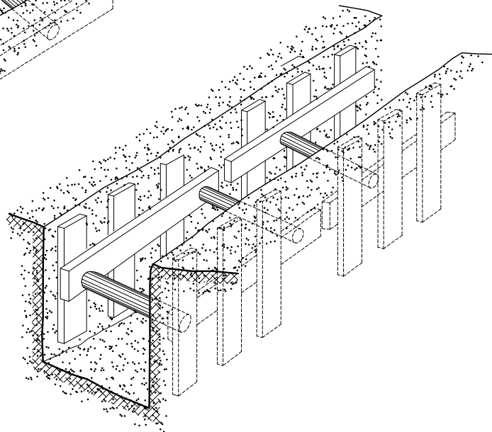
ENTIBACION SEMICUJADA
