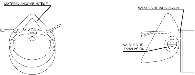
SECCION A-A
