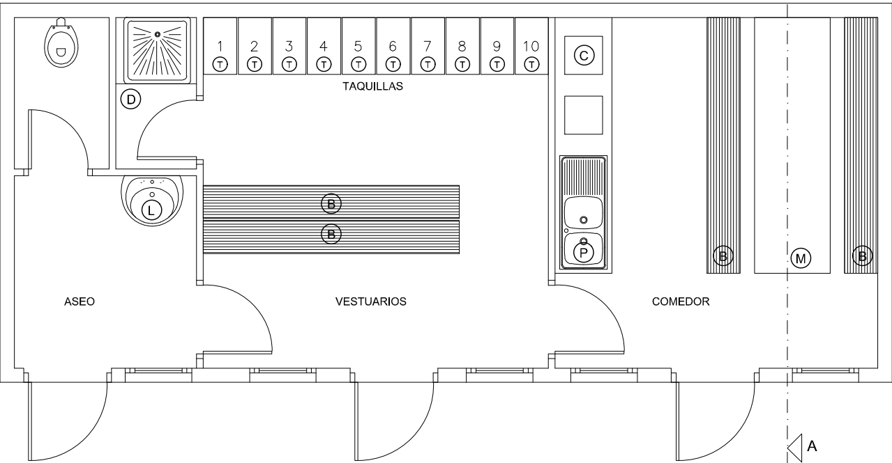
ASEO-VESTUARIOS-COMEDOR MÓDULO TIPO PLANTA
