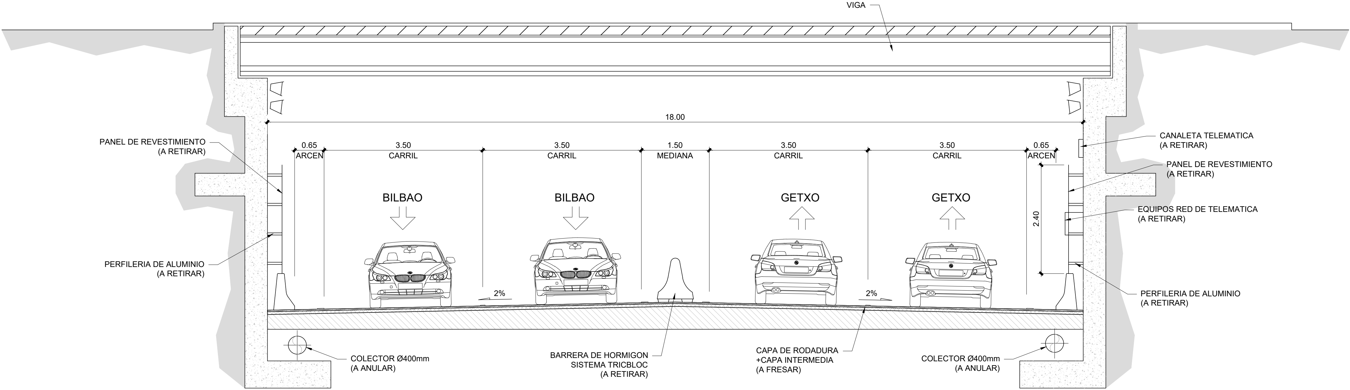
SECCION TIPO ACTUAL BAJO GLORIETAS ESCALA 1/50
