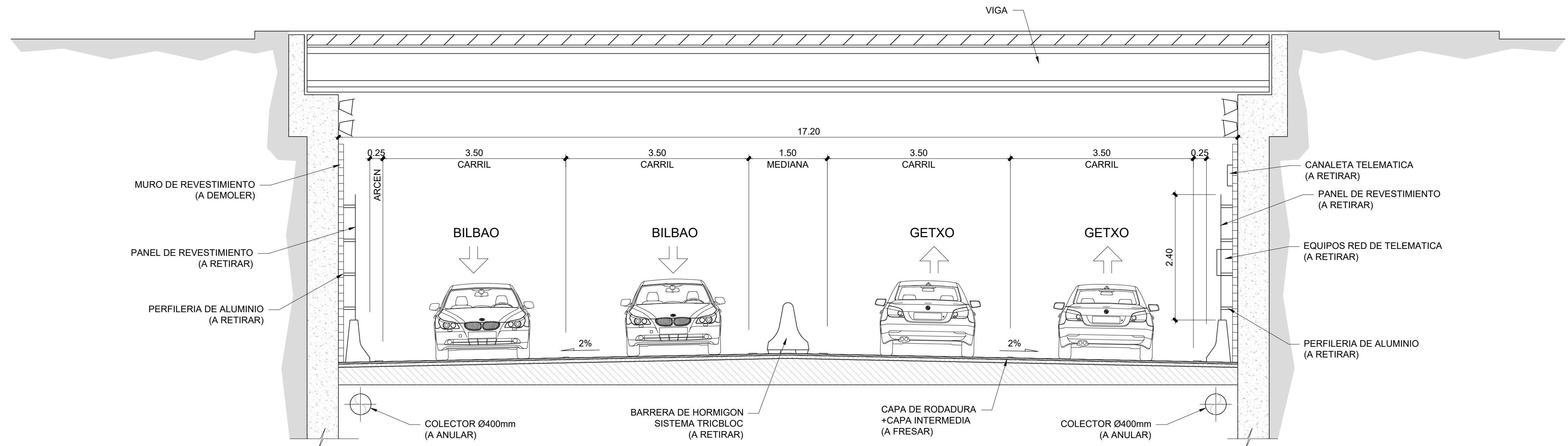
SECCION TIPO ACTUAL DEL FALSO TUNEL DE LA AVANZADA ESCALA 1/50
