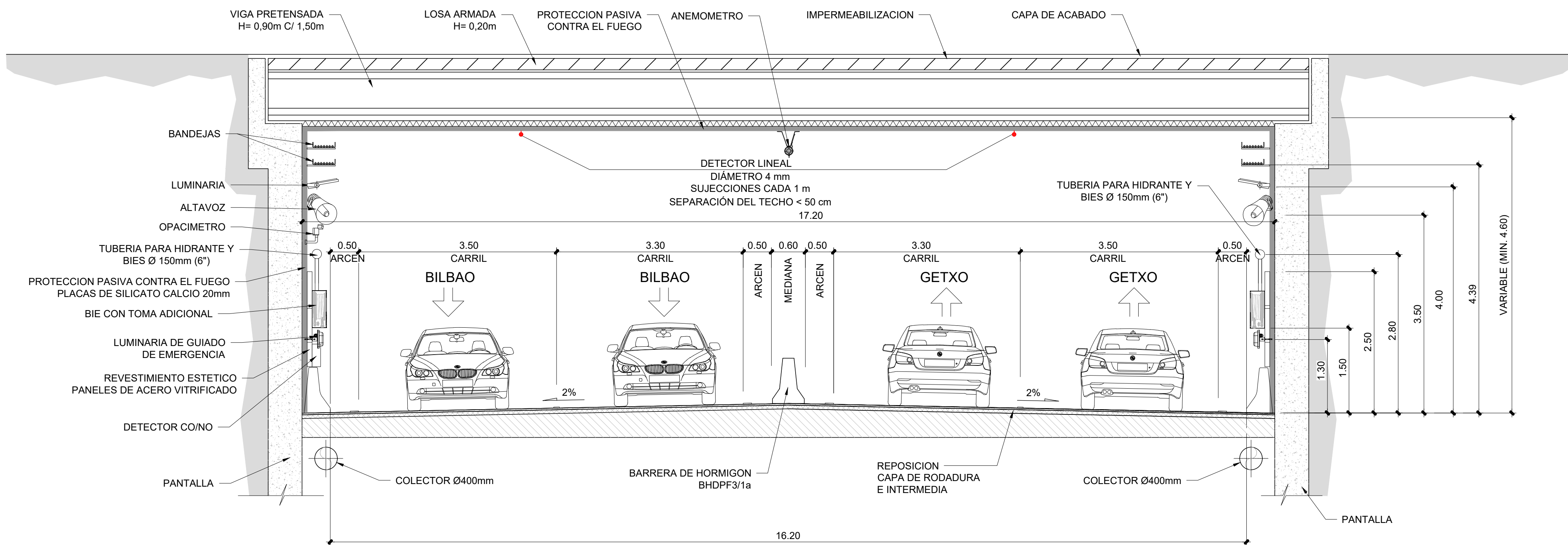
SECCION TIPO PROPUESTA DEL FALSO TUNEL DE LA AVANZADA ESCALA 1/50
