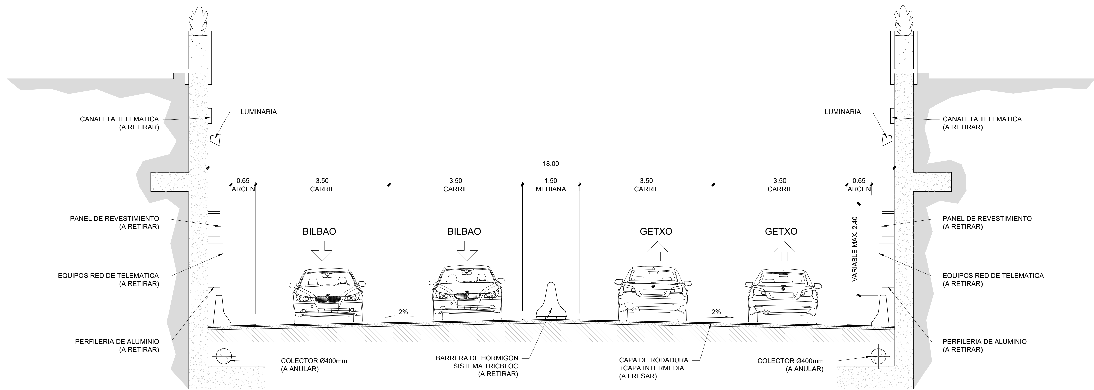
SECCION TIPO ACTUAL ZONA DE TRINCHERA (P.K. 12+256 A 12+386 Y P.K. 12+433 A P.K. 12+511) ESCALA 1/50
