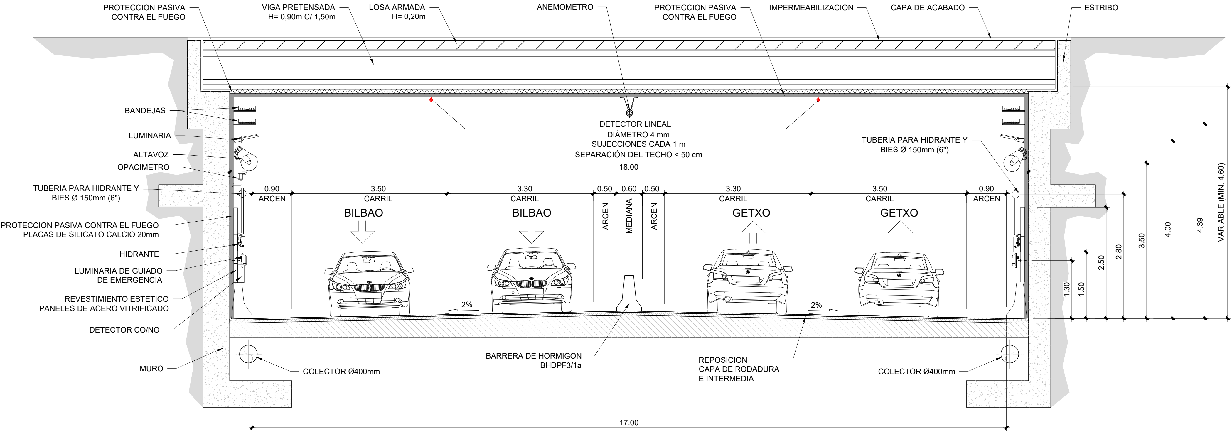
SECCION TIPO PROPUESTA BAJO GLORIETAS ESCALA 1/50
