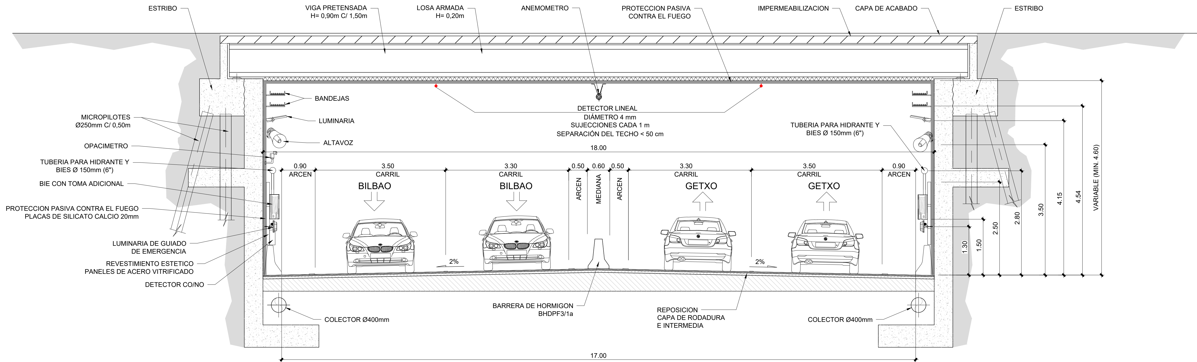
SECCION TIPO PROPUESTA (P.K. 12+256 A 12+386 Y P.K. 12+433 A P.K. 12+511) ESCALA 1/50
