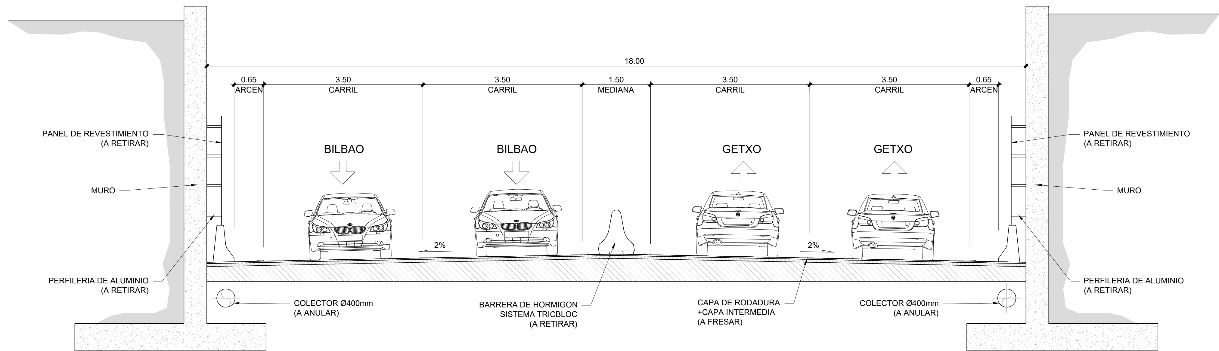
SECCION TIPO TRINCHERA ACTUAL EN ZONAS DE BOCAS ESCALA 1/50
