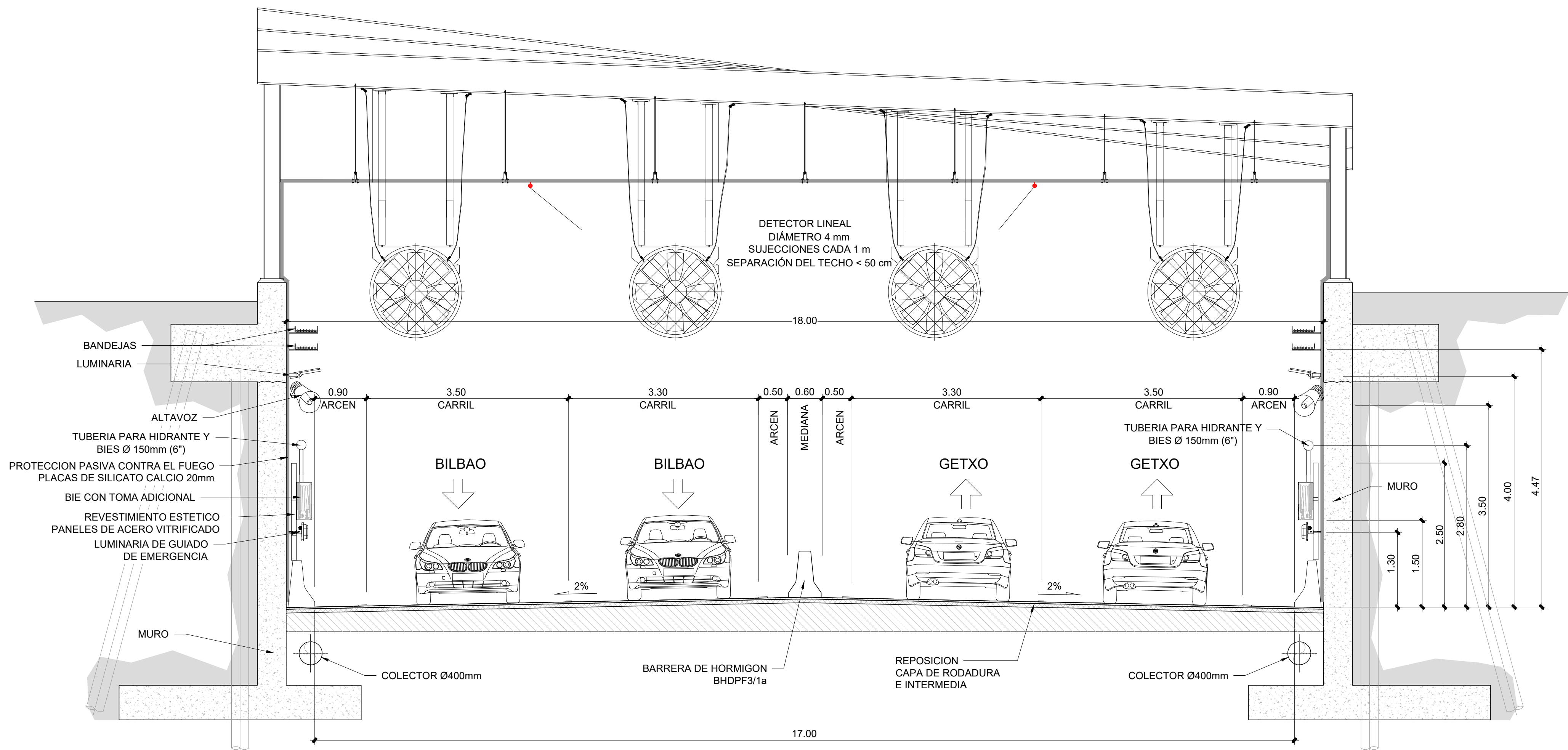
SECCION TIPO TRINCHERA PROPUESTA EN ZONAS DE BOCAS ESCALA 1/50
