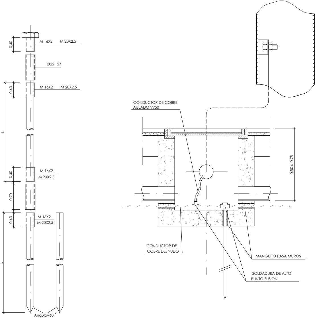
ARQUETA TOMA-TIERRA
