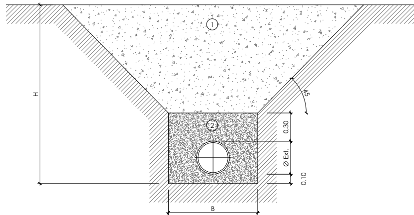
ZANJA TIPO - II SUELO COHESIVO 1,25 < H \leq 2,00
