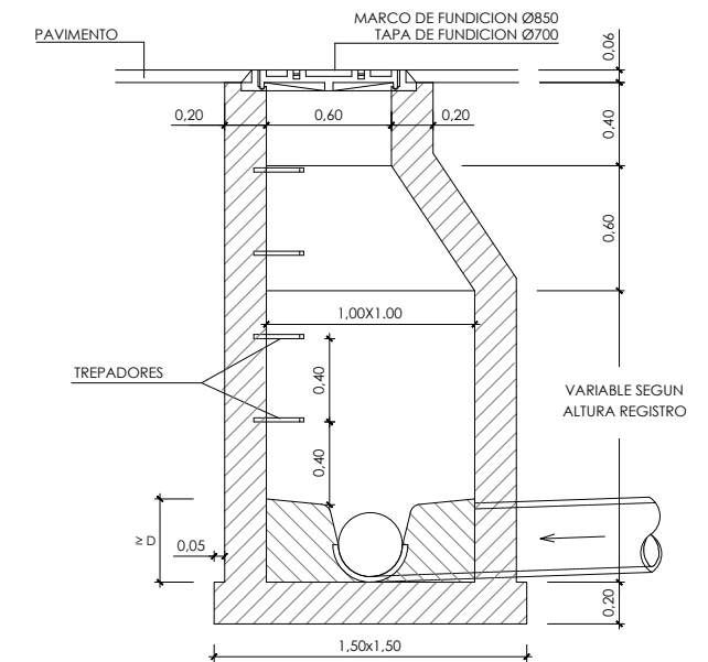
SECCION B-B
