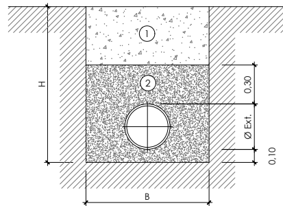
ZANJA TIPO - I SUELO COHESIVO H \leq 1,25
