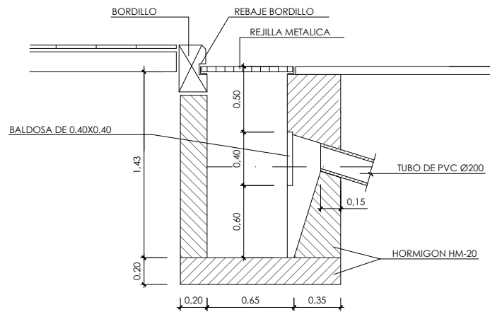
SECCION A-A
