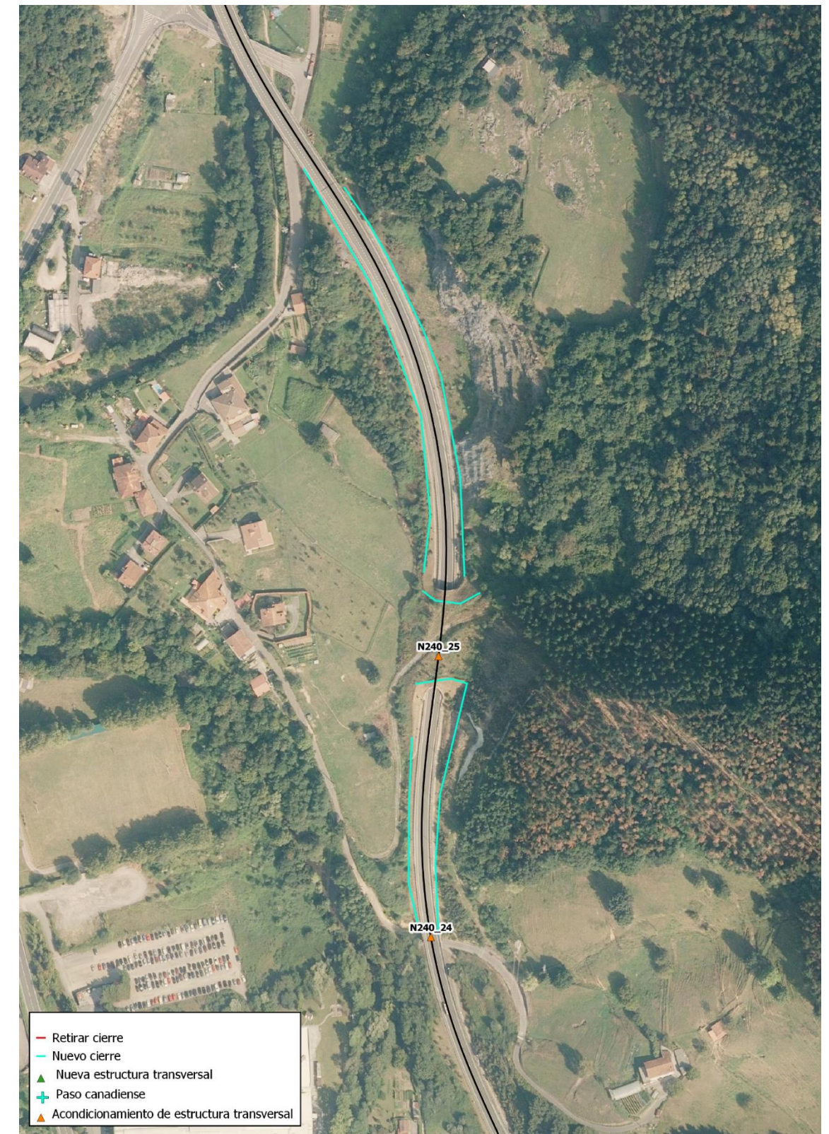
Figura nº44. Actuaciones a realizar en el tramo Lemoa – Igorre
