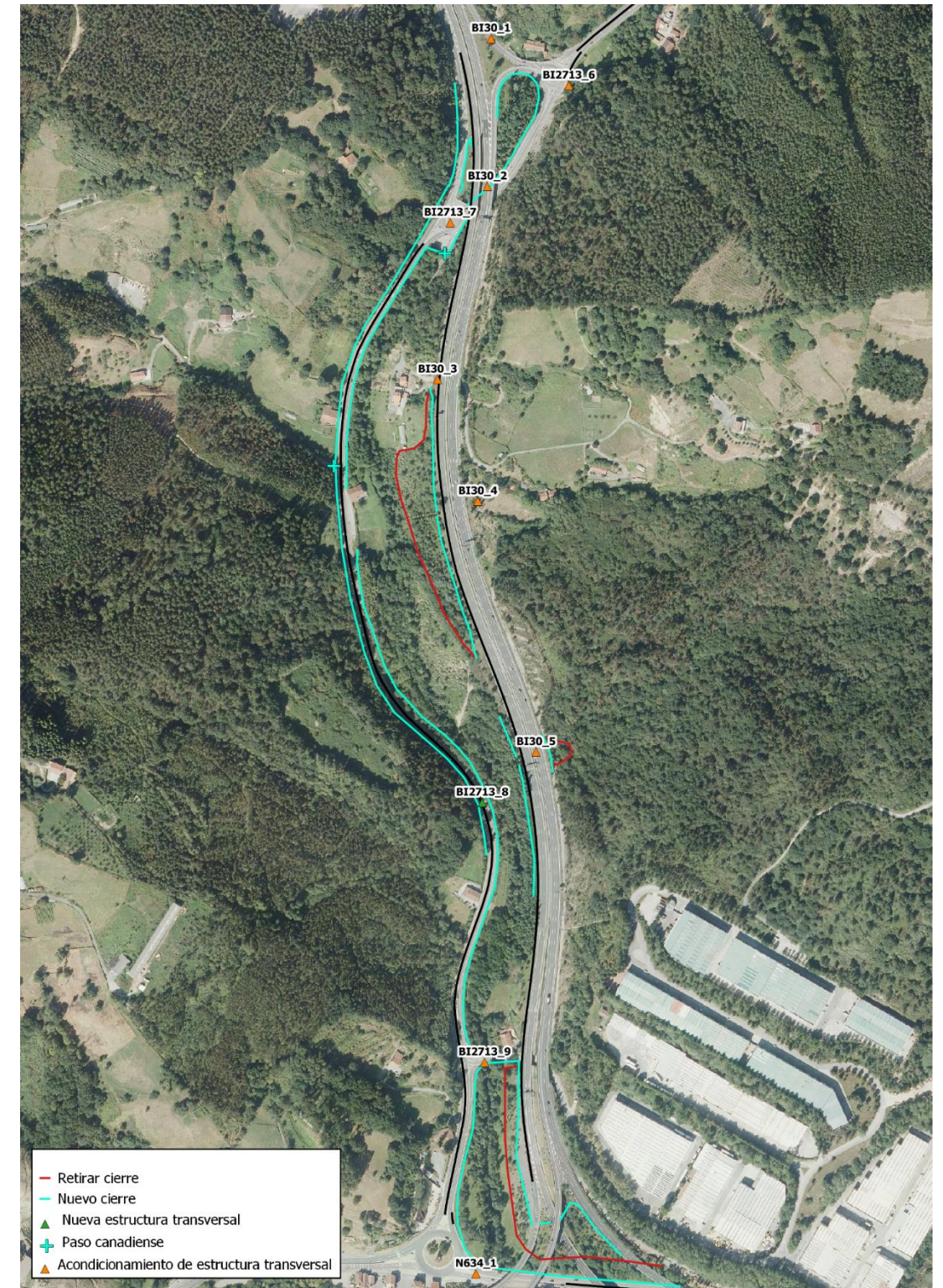
Figura nº13. Actuaciones a realizar en el tramo de Alto de Morga – BI-2121.
