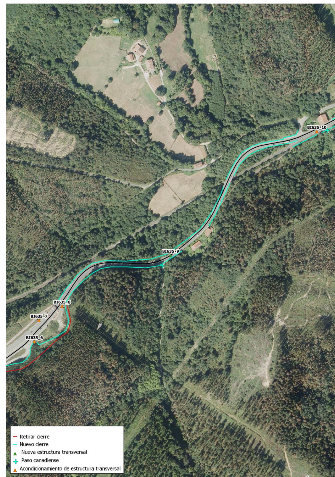
Actuaciones a realizar en el tramo Final túnel de Autzagane - Gorozika.
