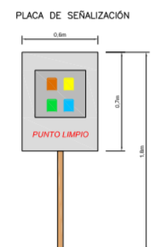
Plano nº 4 Detalle cubierta recinto residuos peligrosos y placa señalización punto limpio.
