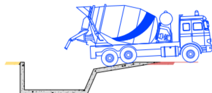
Plano nº 6 Detalle punto de limpieza canaletas de las hormigoneras.
