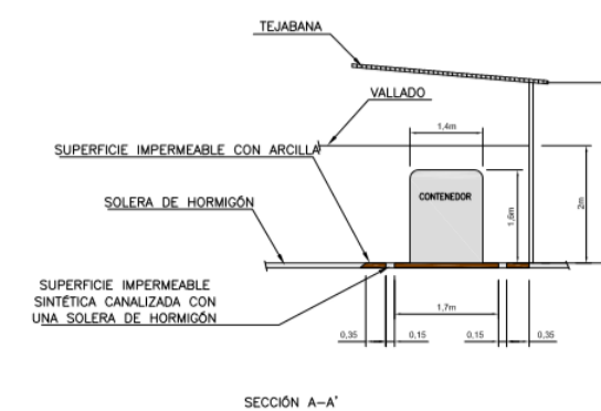
Plano nº 4 Detalle cubierta recinto residuos peligrosos y placa señalización punto limpio.
