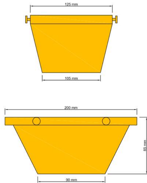
Plano nº 5 Detalle contenedor tipo R.C.D.
