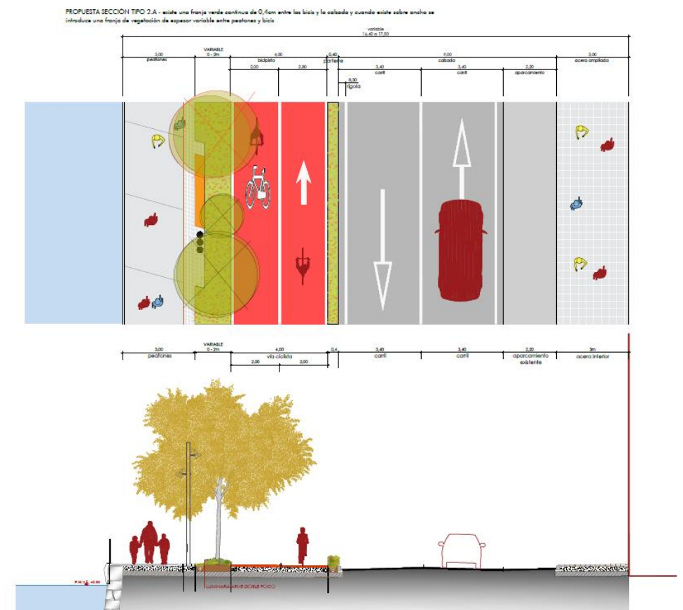
SITUACION TIPO DEL PASEO CON POSIBILIDAD DE SOBRECARGO PARA ZONAS VERDES O ESTANCIALES
