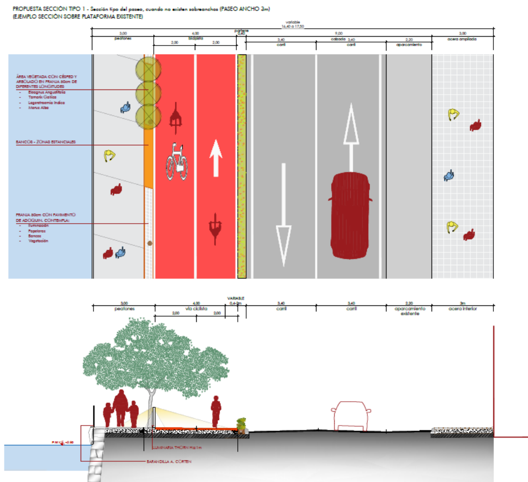
SITUACION TIPO DEL PASEO DE 3 M
