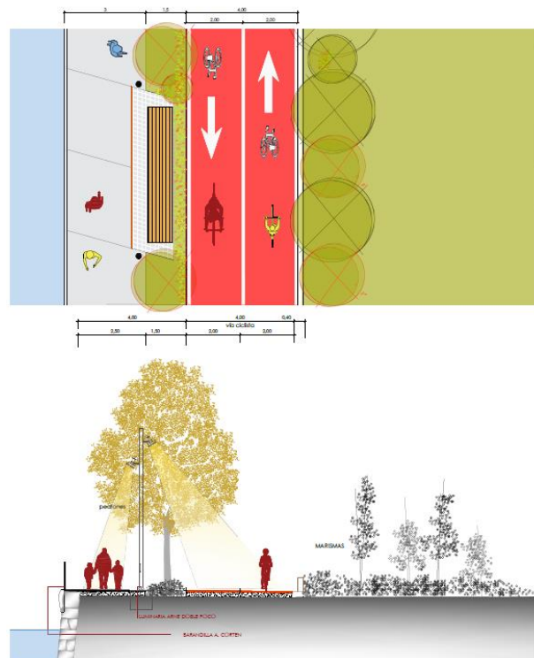
PROPUESTA SECCIÓN TIPO 4 -MÁRSHAS DE LANIAKO ZONAS MÁS ESTRECHAS (FASEO PEATONAL DE 4,5m)
