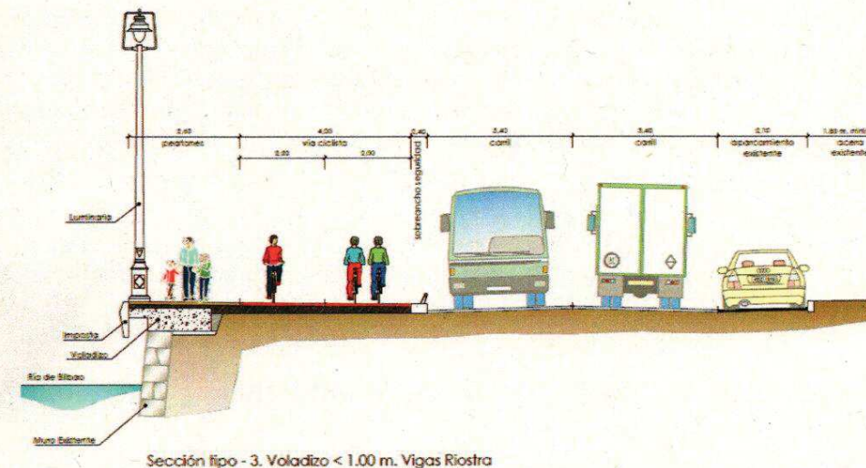
Sección tipo - 3. Voladizo < 1.00 m. Vigas Rostro
