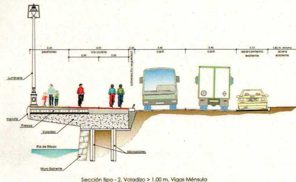
Sección tipo - 2. Voladizo > 1.00 m. Vigas Ménsula
