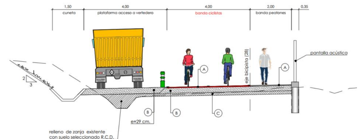
ST-15 Senda ciclable y peatonal sobre pista con desmonte
