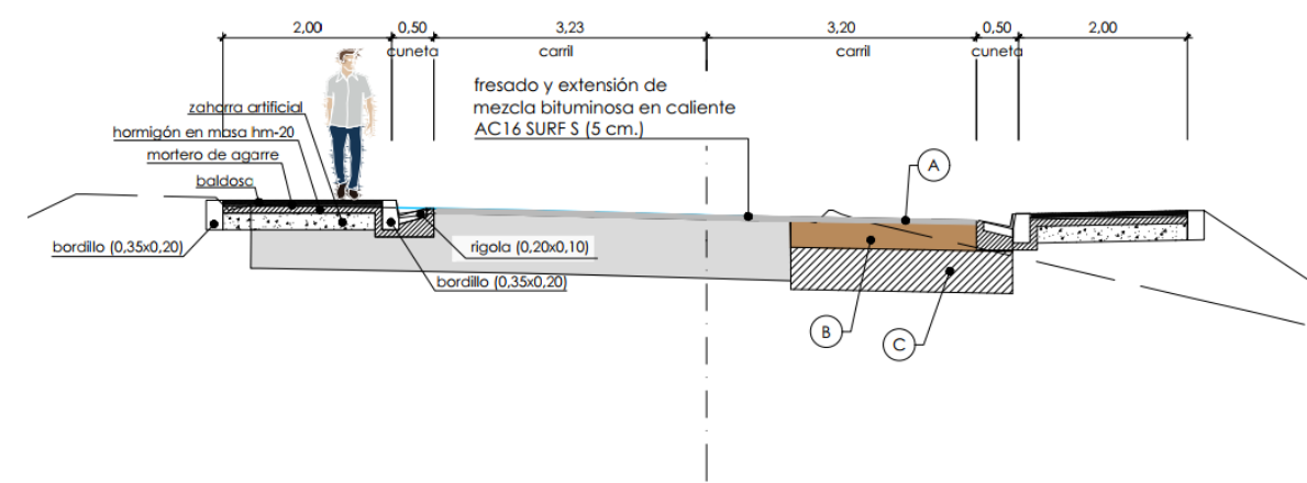
Reposición vial acceso Este polígono Erletxe (eje 26)
