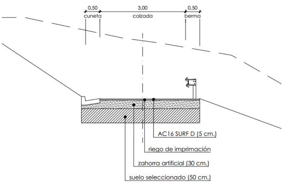
Reposición camino 4+300 (eje 29)
