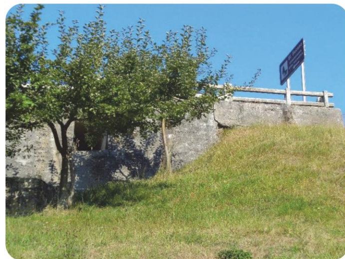
50+660 Muro de hormigon en MI -9
