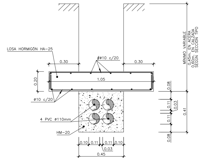
ZANJA TIPO CON LOSA PARA 4 PVC Ø110mm ESCALA 1/10
