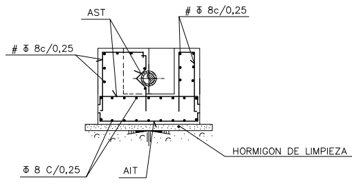
SECCION F-F
