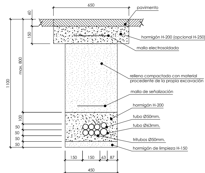
Construcción de canalización en asfalto tipo 7 hasta 1,1m. de profundidad (2 tritubos de 50mm., 1 tubo de 63mm. y un tubo de 50mm.) Escala 1:10
