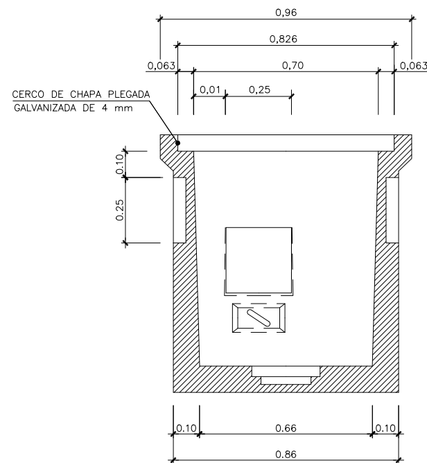
SECCION B-B
