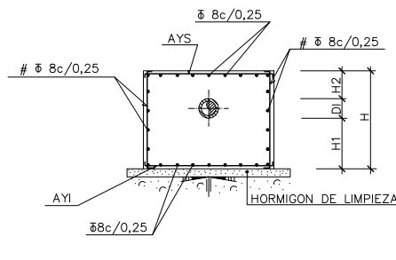
SECCION C-C
