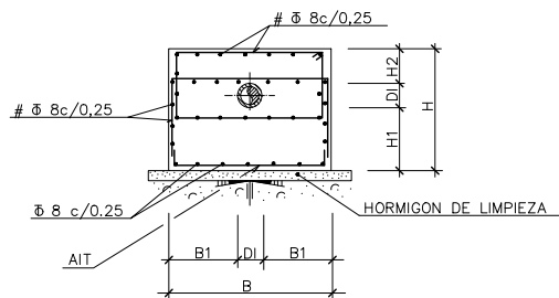
SECCION E-E
