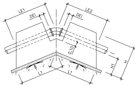
ANCLAJE TIPO EN ALZADO-CONVEXO FORMAS
