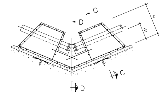
ANCLAJE TIPO EN ALZADO-CONCAVO ARMADURAS
