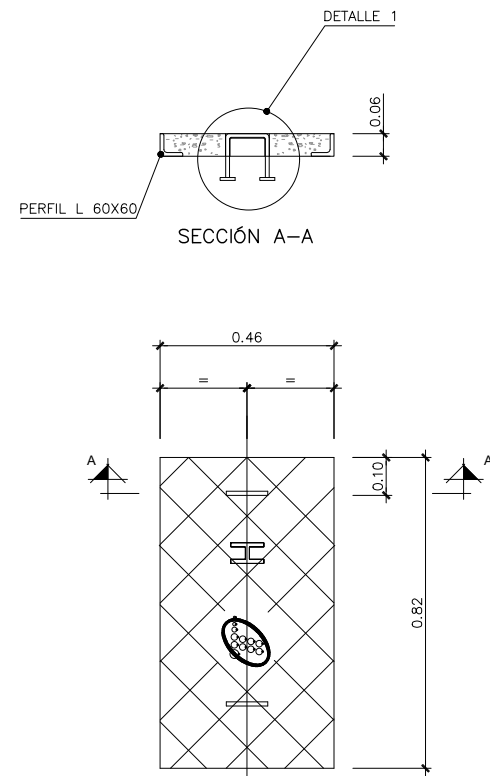
PLANTA
