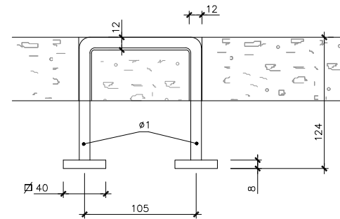
DETALLE 1 ASA DE LEVANTAMIENTO DE TAPA ESCALA 1/2.5 (COTAS EN mm)
