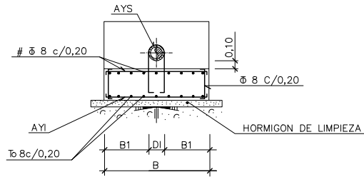
SECCION B-B
