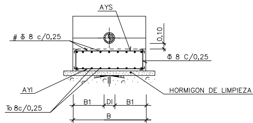
SECCION D-D
