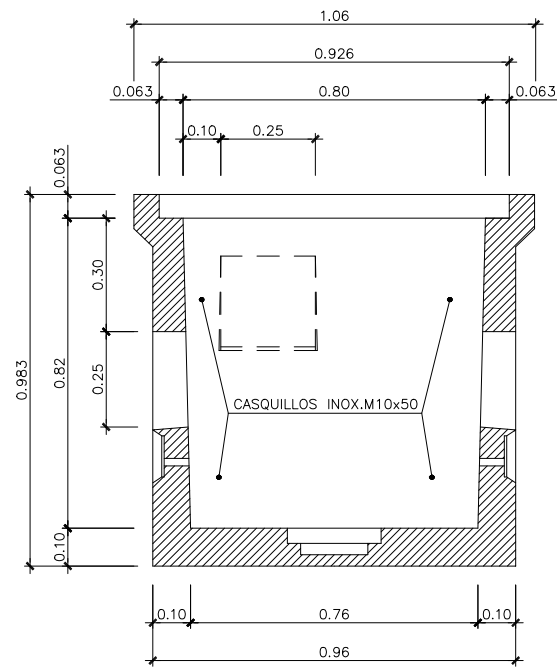
SECCION A-A
