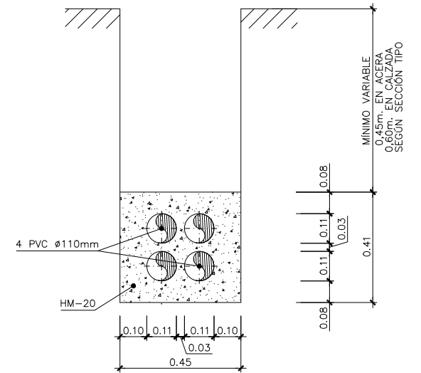
ZANJA TIPO PARA 4 PVC Ø110mm ESCALA 1/10
