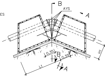
ANCLAJE TIPO EN ALZADO-CONVEXO ARMADURAS
