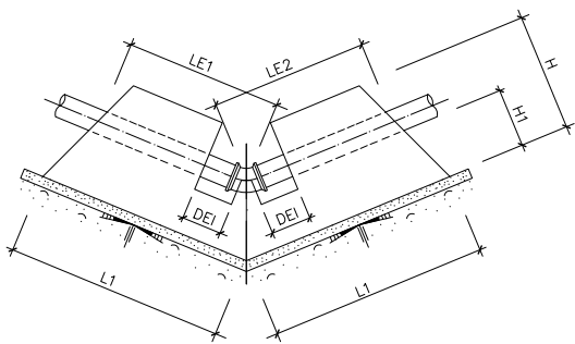
ANCLAJE TIPO EN ALZADO-CONCAVO FORMAS
