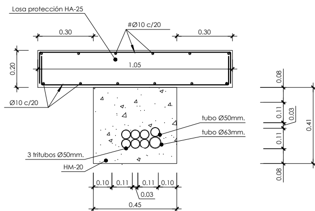
CONSTRUCCIÓN DE CANALIZACIÓN CON LOSA PARA 4 PVC Ø110mm ESCALA 1/10
