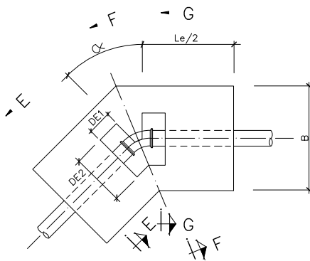
ANCLAJE TIPO EN PLANTA FORMAS
