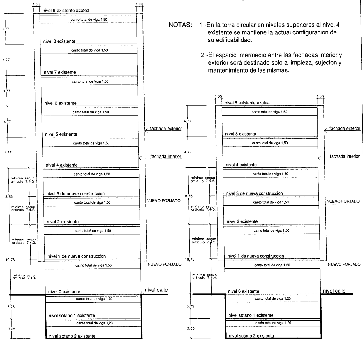
PERFIL A EN TORRE CIRCULAR
